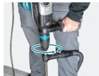
Za siguran rad obavezno držite crijevo usisivača rukom ili ga naslonite na nogu da sprečite uvrtanje.
